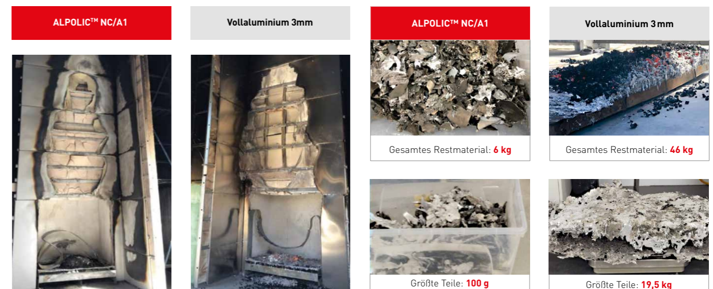
Ergebnis nach einem Großbrandtest (BS8414-2)
